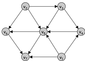
a DAG
