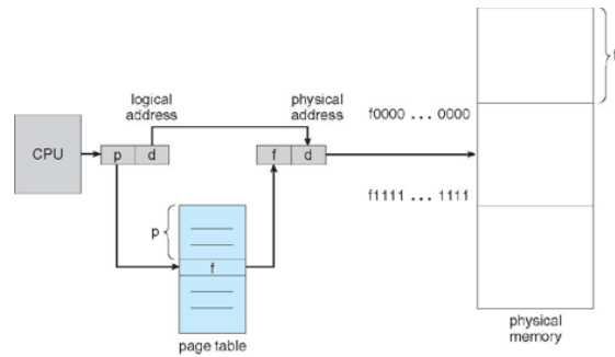
Paging without TLB
